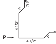
F Gutter Apron TLGA29 10'2"
